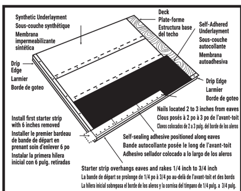
Figura A: Instalación de la tira de arranque
